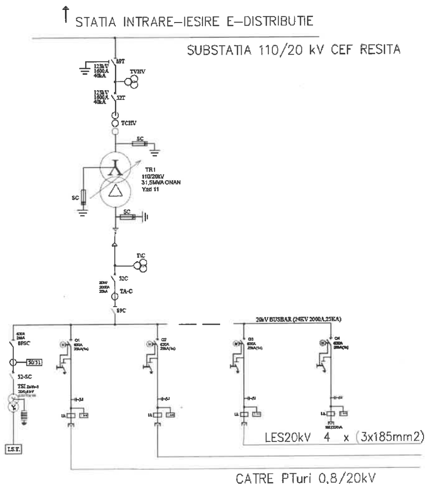
Figură 3.18 Schemă monofilară a stației 110/20 kV de evacuare a puterii CFE
