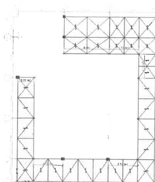
Plan planșeu și structură metalică cota +11.20 m
