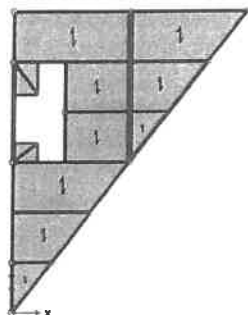
Plan planșeu compozit cota +4.65 m
